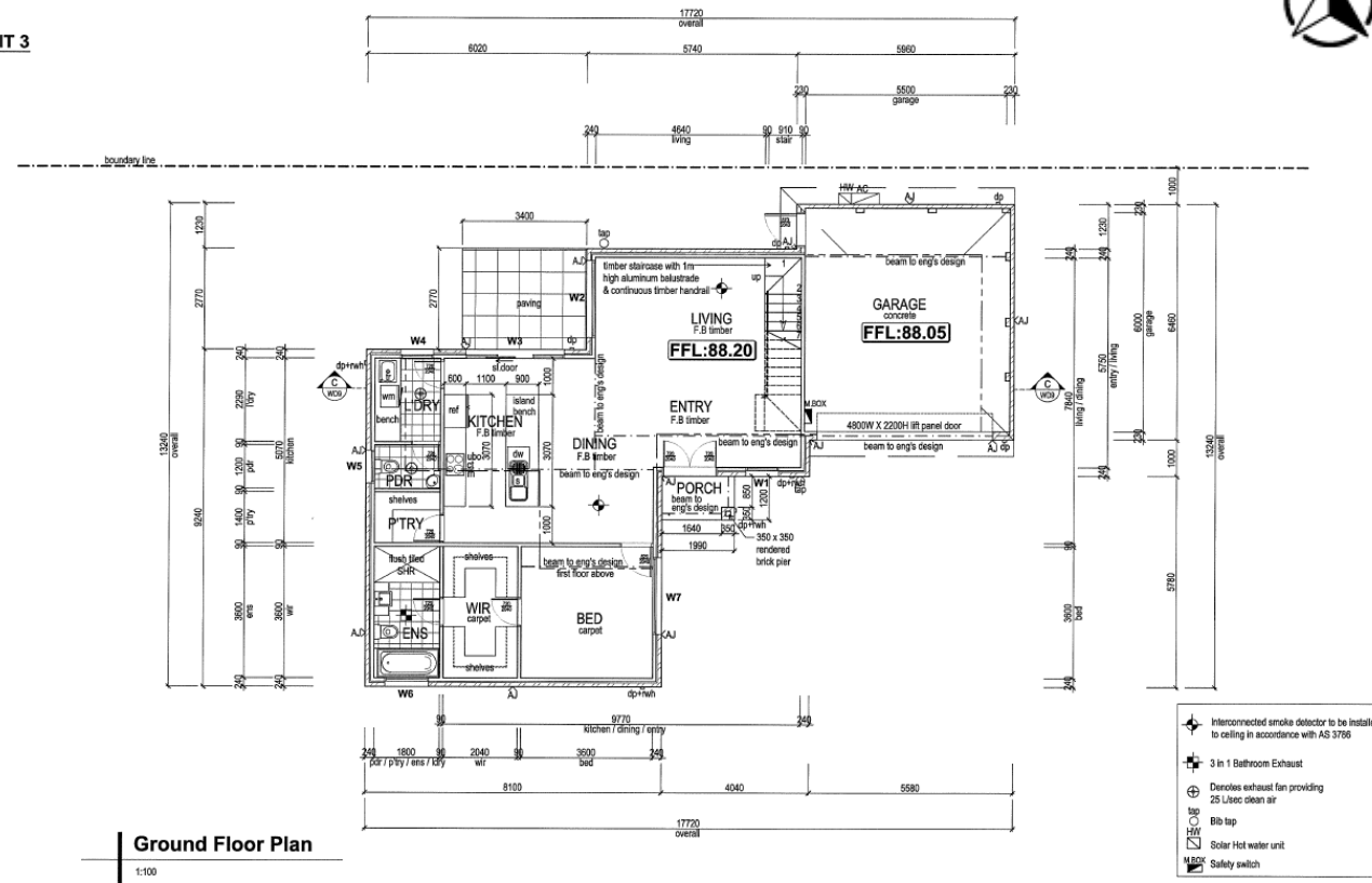
首层平面图
